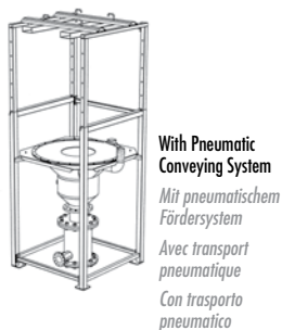
With Rotary Valve Mit Zellenradschleuse Avec sas alvéolaire Con rotovalvola
